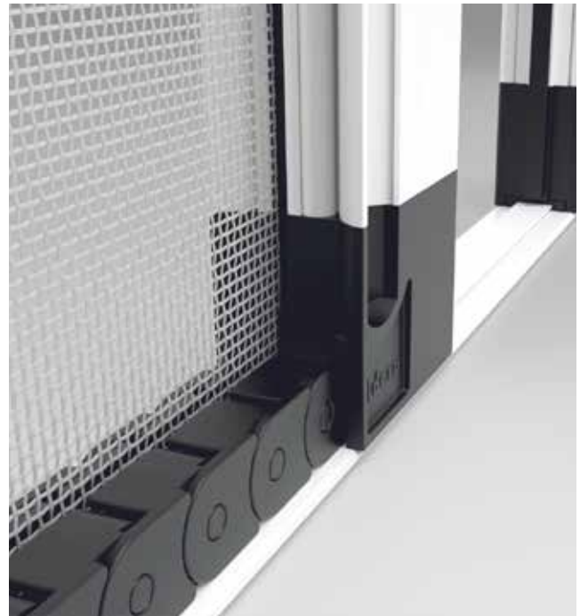
Unterer Teil der Gleitführung
