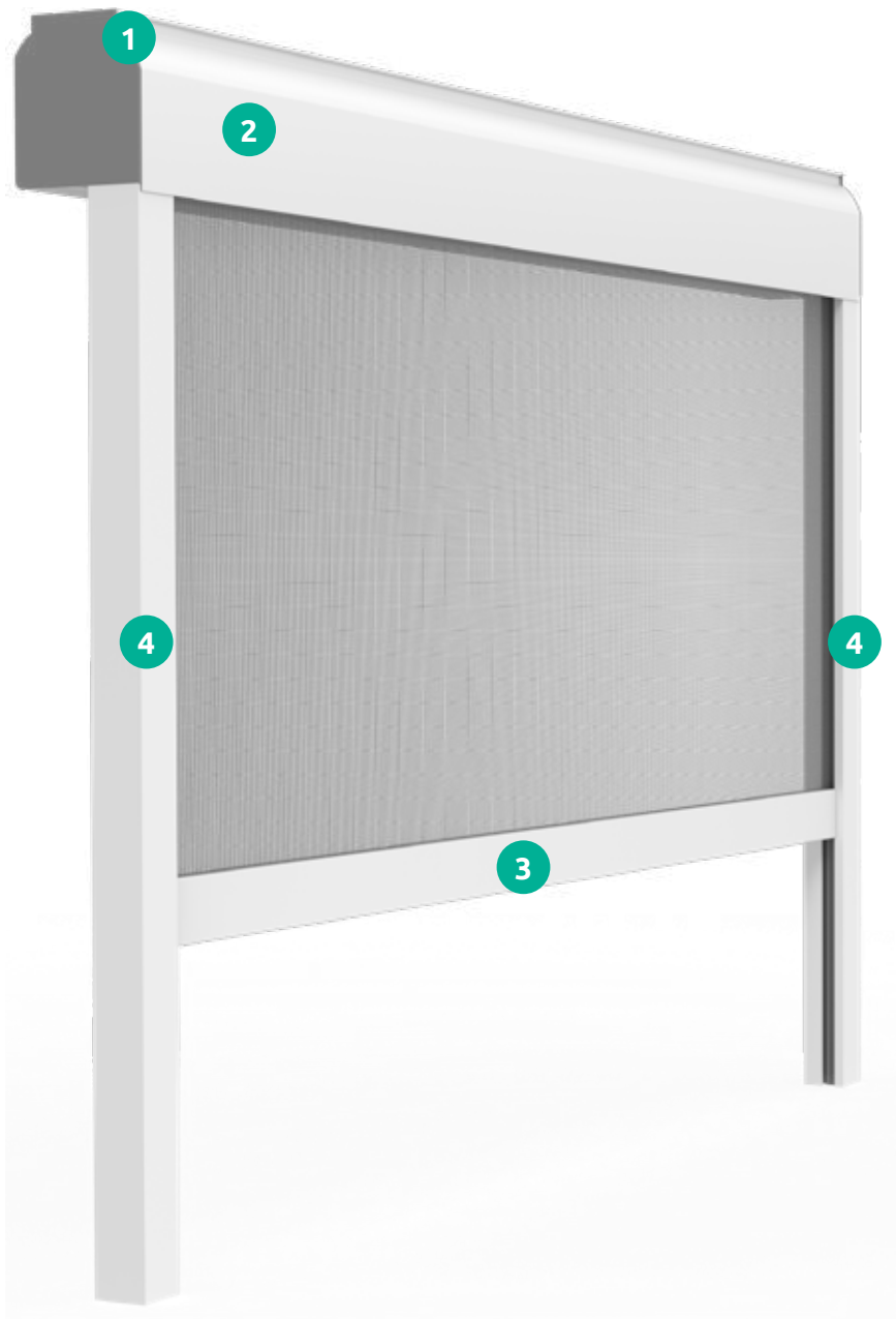
1 Gehäuse-Haltevorrichtung
