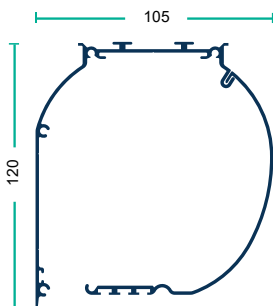
2 Gehäuse
