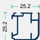
2 Montagerahmenprofil
