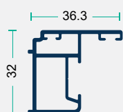
1 Drehtüreprofil
