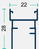
01 Deckenprofil
